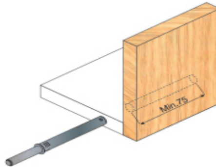
Pulsador Ø10 largo
