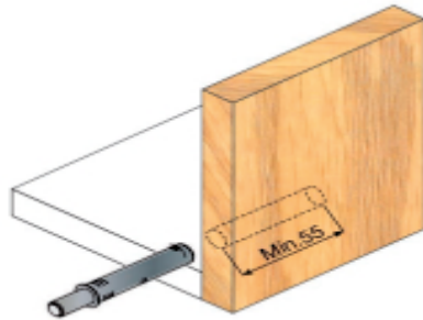
Pulsador Ø10 curto
