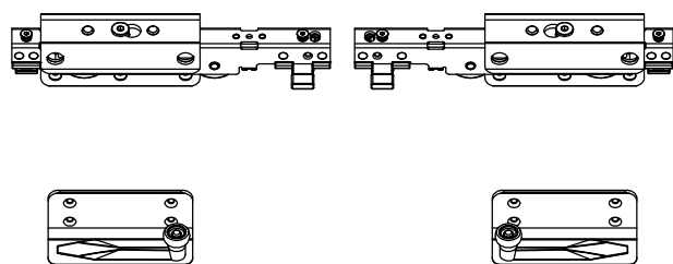
Running part and guiding part of inner door /Lauf- und Führungswagen Türe innen
