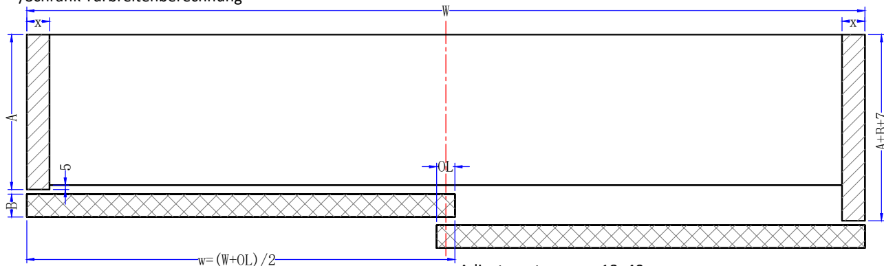
Cabinet door width calculation /Schrank Türbreitenberechnung
