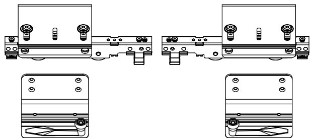
Damper /Dämpfer
